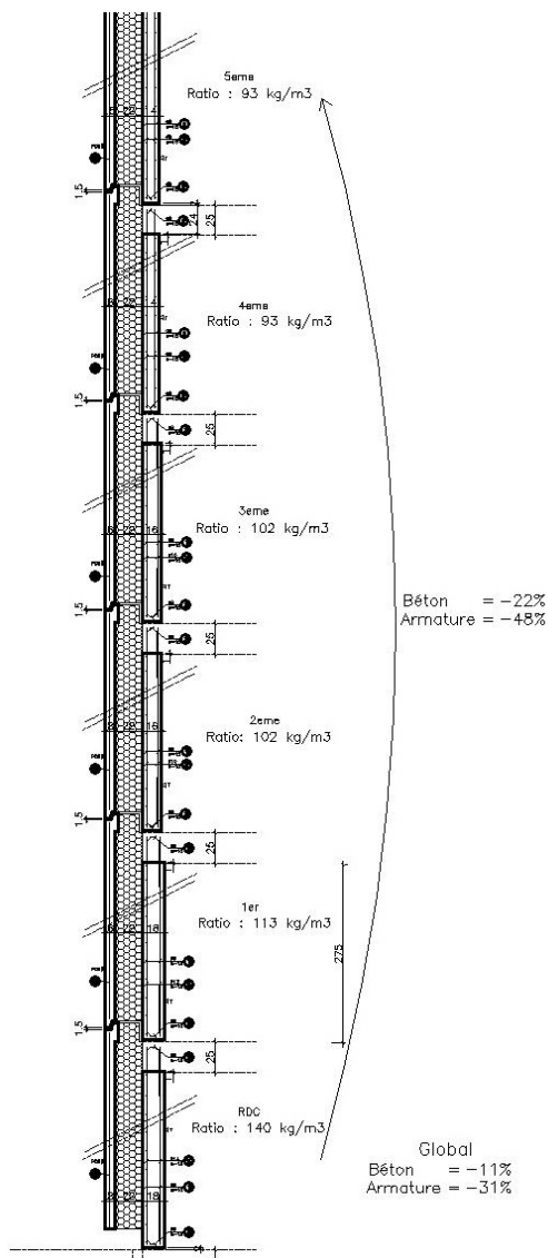
Optimisation du taux d'armature et des épaisseurs de la façade porteuse PRELCO
