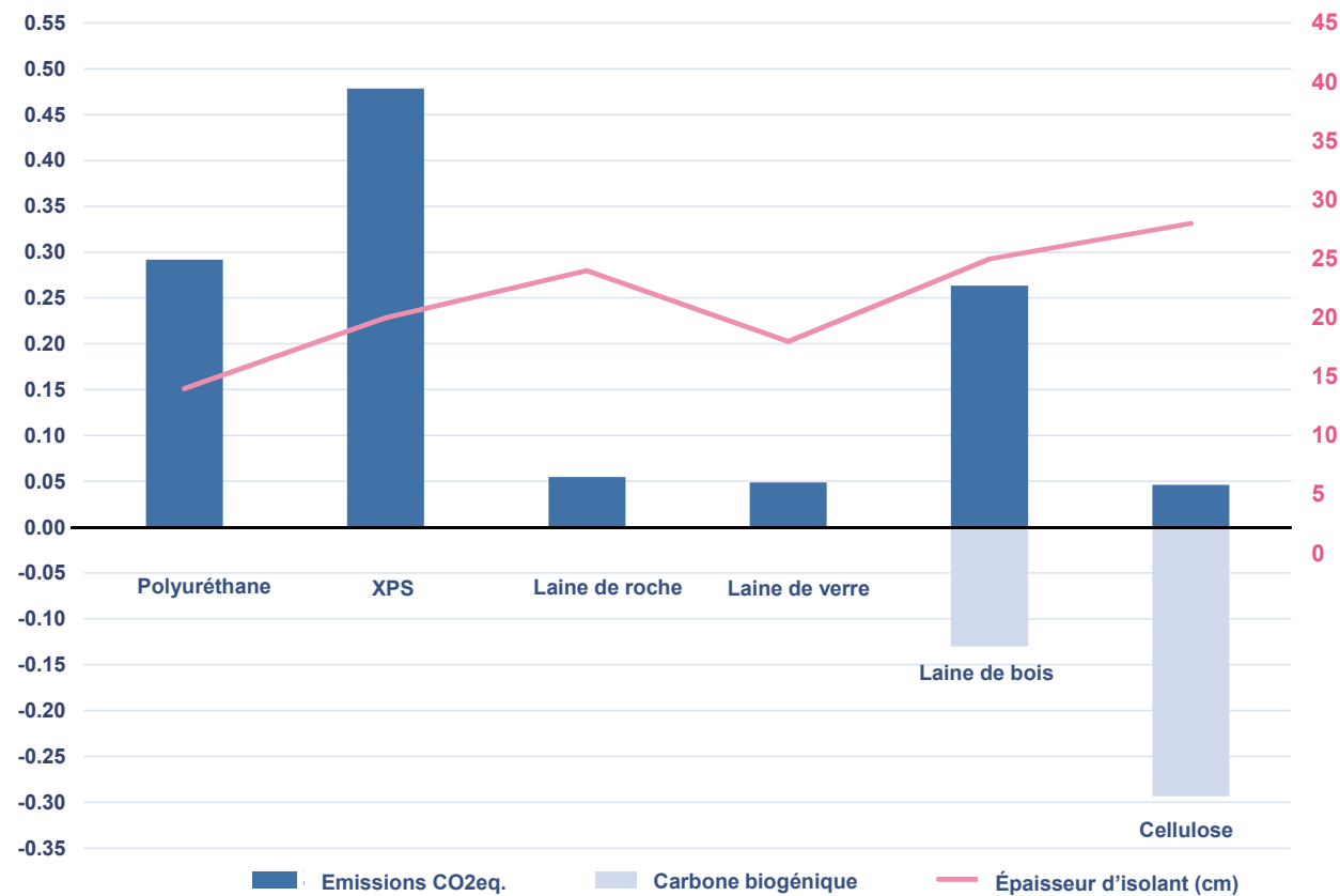
Variation de l'isolant de la façade PRELCO sur le bâtiment référence ( U=0.15 \text{ W/m}^2\text{K} ) \text{KgCO}_2/\text{m}^2\text{a}
