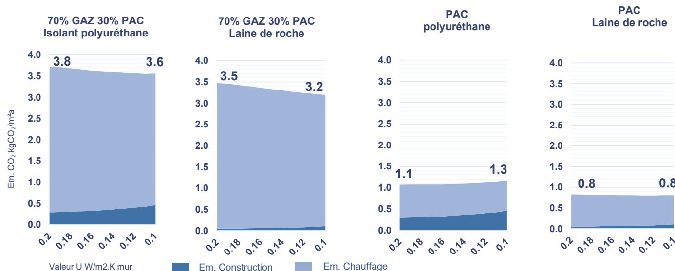
Étude de influence de l'épaisseur d'isolant et du type de vecteur énergétique sur les émissions carbone directes et indirectes du bâtiment de logement
