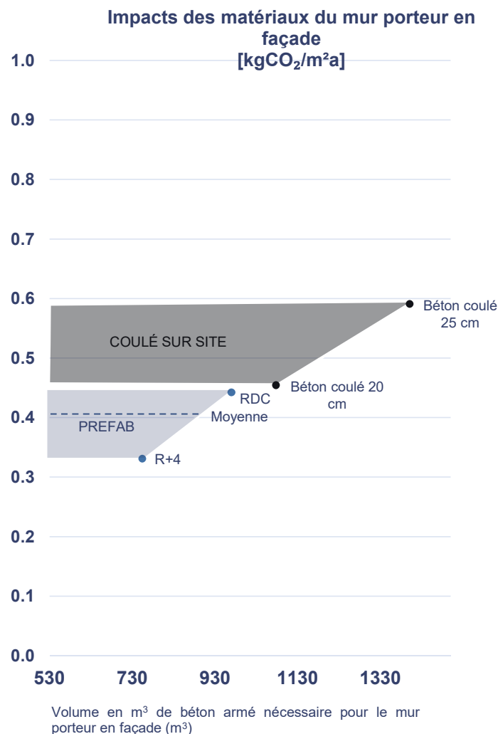
Étude de l'influence de l'épaisseur et du taux d'armature du mur porteur en façade sur les impacts du projet de référence
