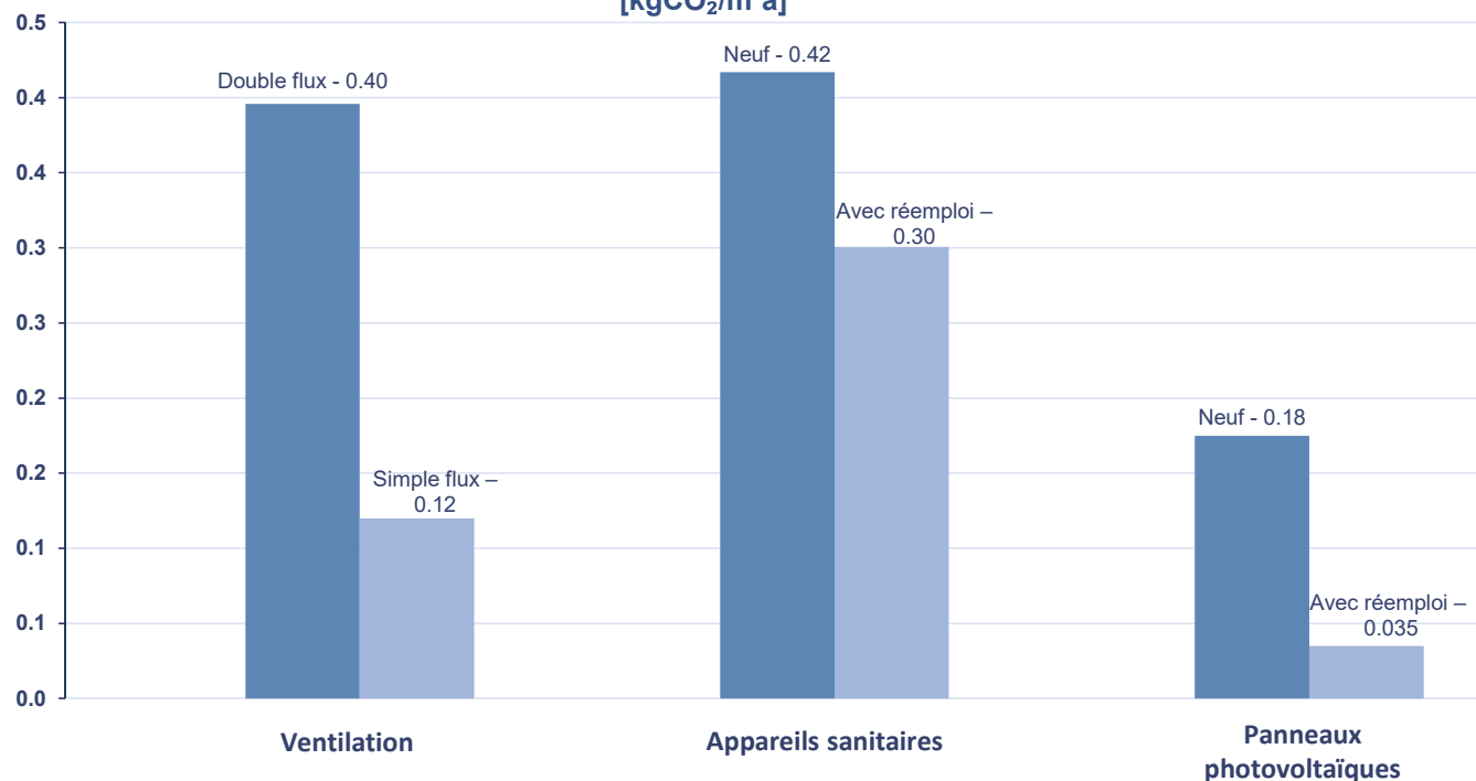
Impact des optimisations des installations sur le bâtiment de référence [kgCO 2 /m 2 a]
