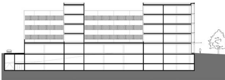
Coupe longitudinale
